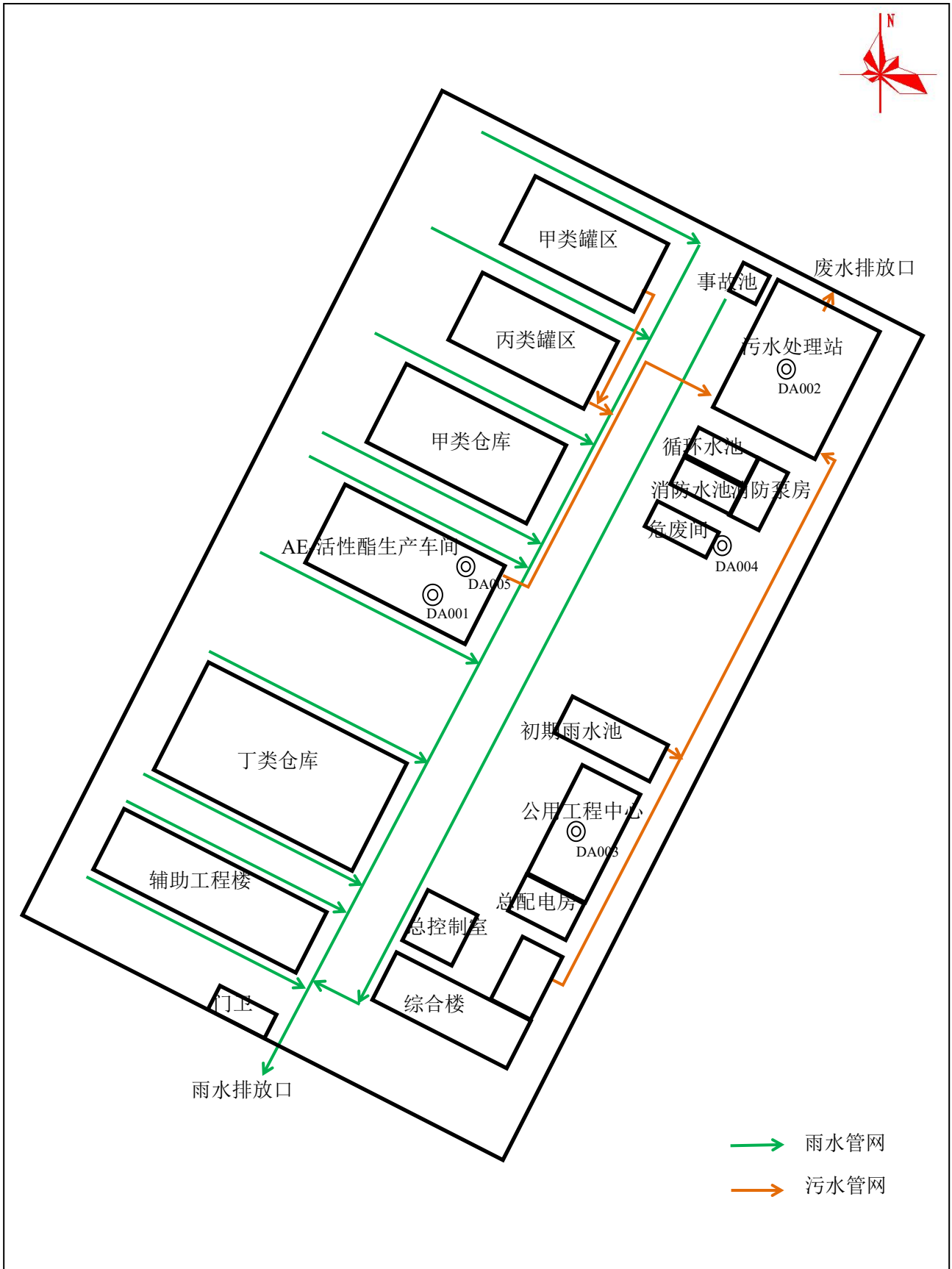
附图 4 项目雨污管网图
